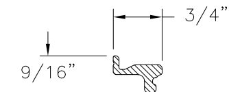
STILE LINER FIBERGLASS (MS400320)
