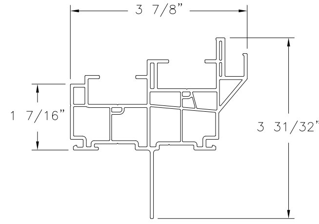
JAMB FRAME FIN INSTALLATION RIGID PVC (V-1033)
