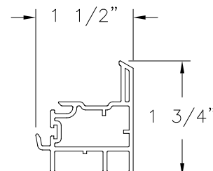
BOTTOM SASH TOP RAIL RIGID PVC (V-675)
