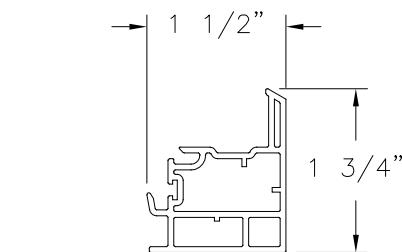
BOTTOM SASH TOP RAIL RIGID PVC (V-675)
