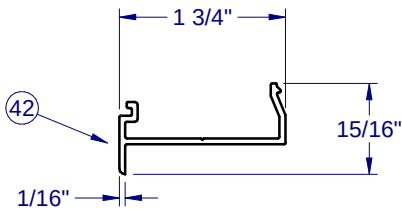
Screen, Astragal - 2137
