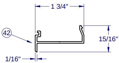
Screen, Astragal - 2137
