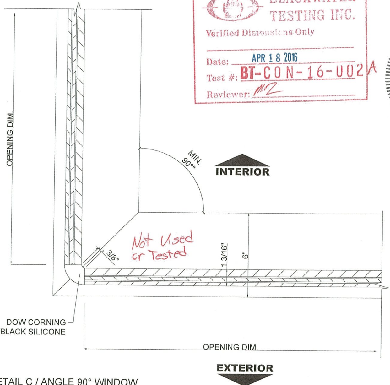
DETAIL C / ANGLE 90° WINDOW SCALE: 3"=1'-0"
