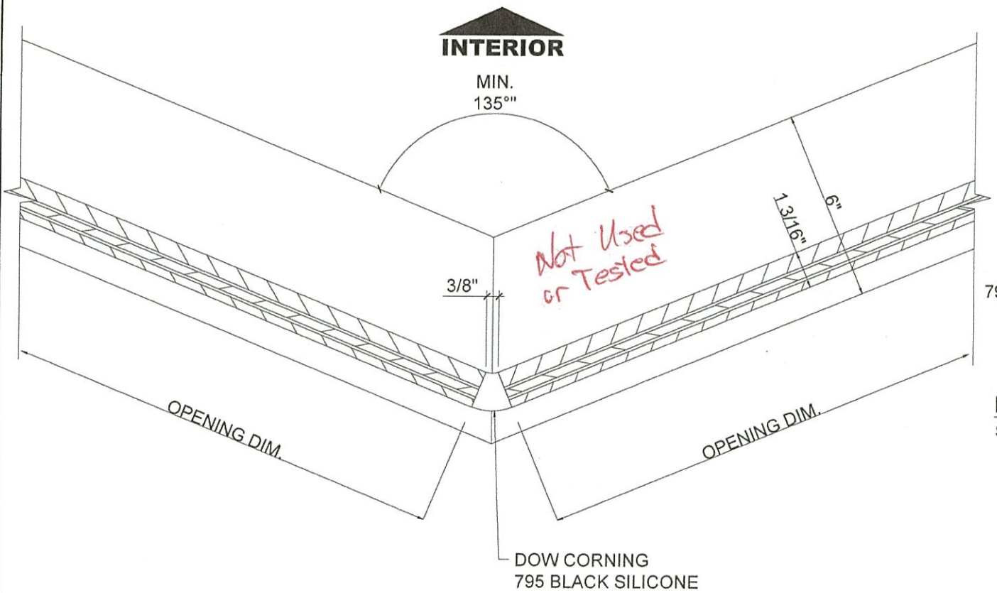
DETAIL B / NEO-ANGLE WINDOW SCALE: 3"=1'-0"
