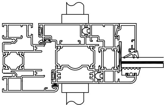
locking left side jamb
