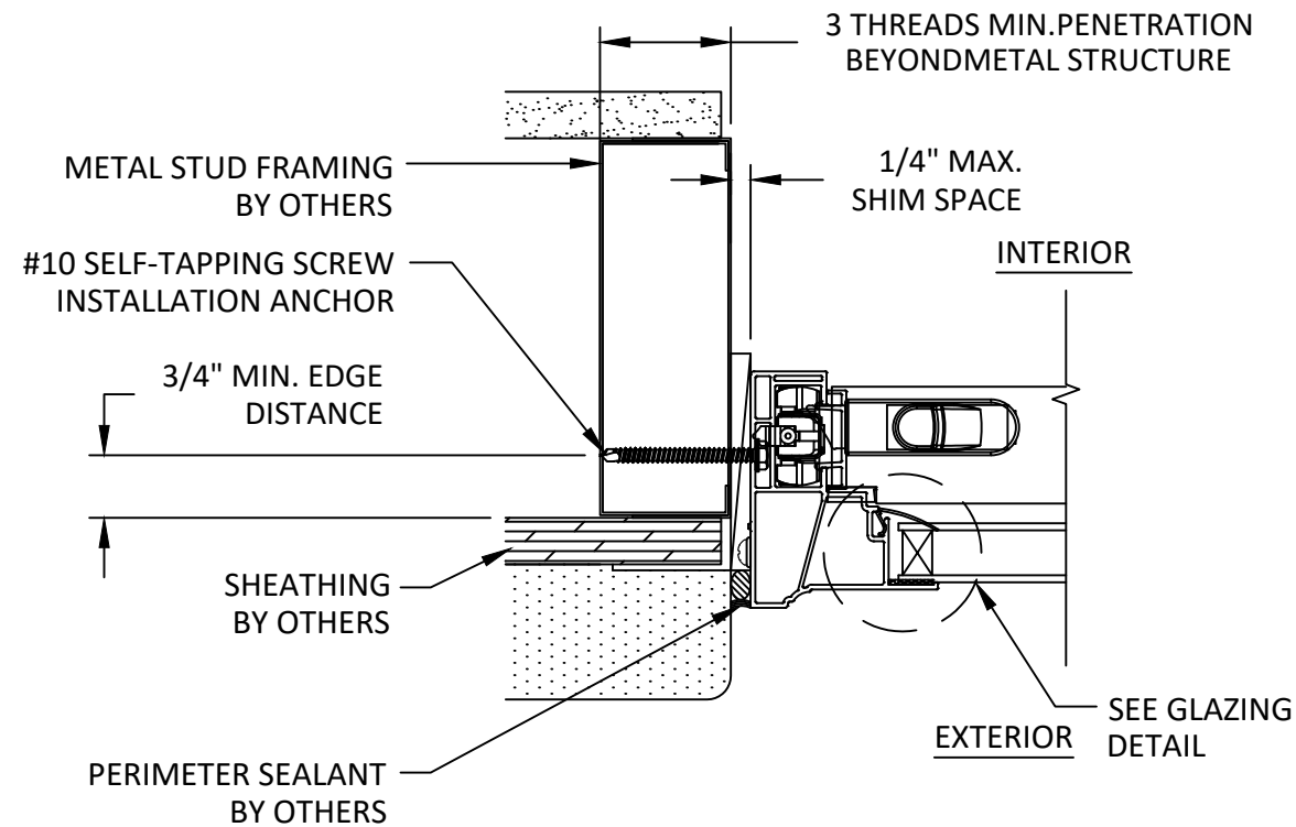
F5 HORIZONTAL SECTION SINGLE HUNG JAMB - METAL STUD FRAME
