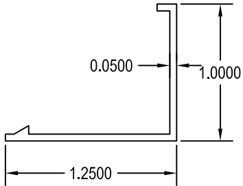
5 #36 TRIM SCALE 1:1
