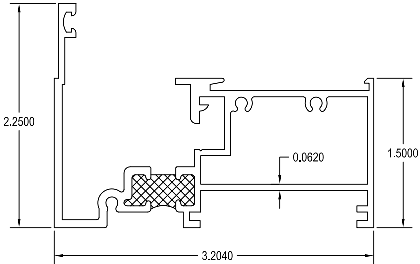
2 FRAME SILL SCALE 1:1
