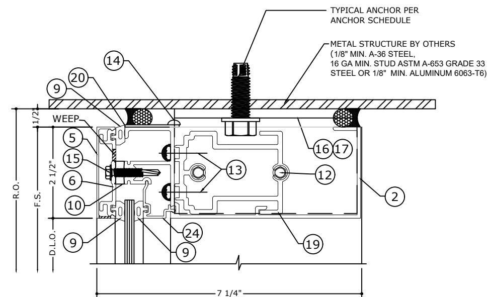
1.5 HEAD DETAIL SCALE: 6" = 1'-0"
