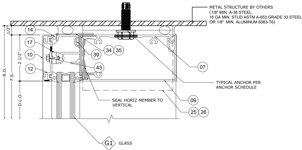
1.2 HEAD DETAIL SCALE: 6" = 1'-0"
