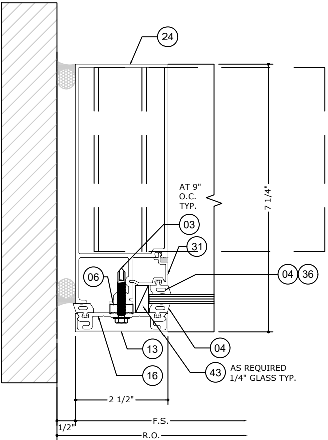
4.1 JAMB DETAIL SCALE: 6" = 1'-0"
