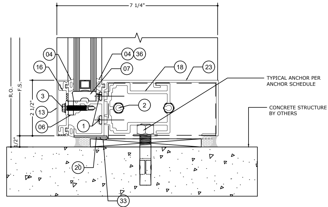
2 SILL DETAIL SCALE: 6" = 1'-0"
