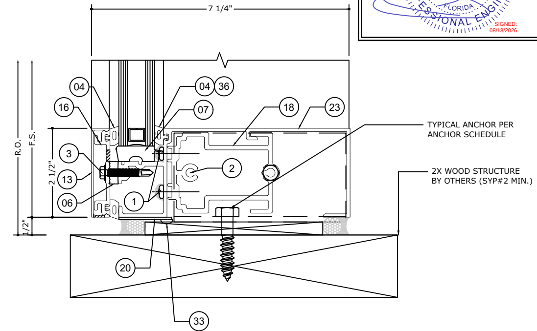
2.1 SILL DETAIL SCALE: 6" = 1'-0"
