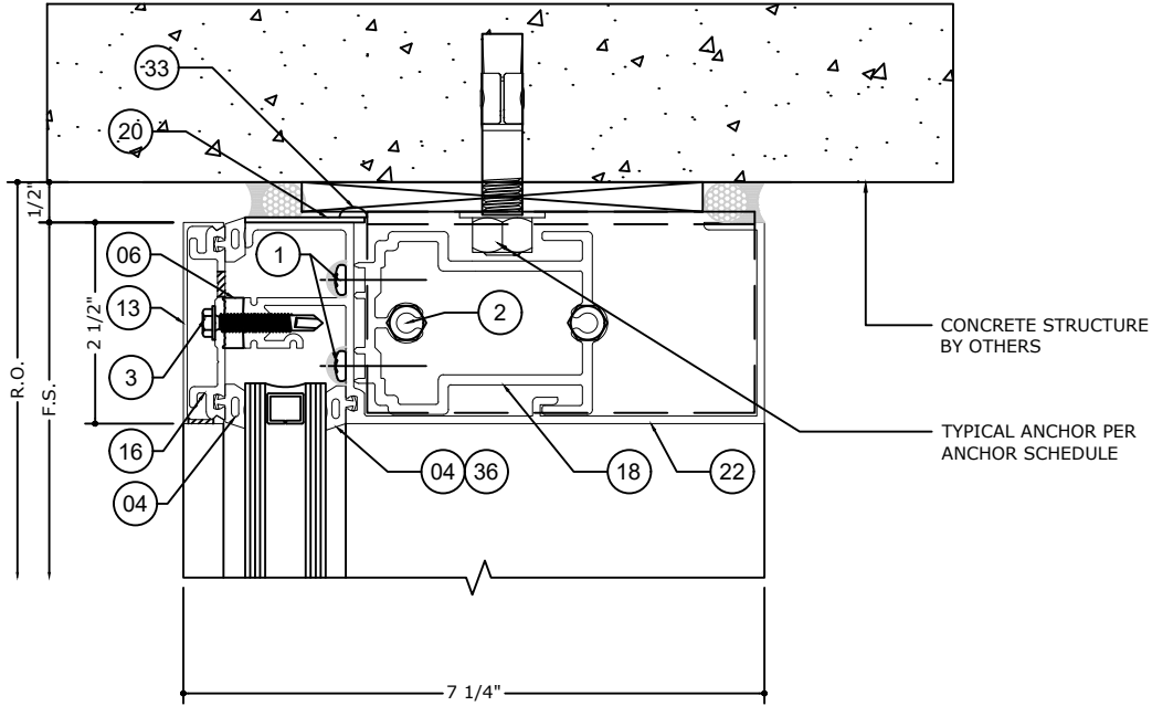
1 HEAD DETAIL SCALE: 6" = 1'-0"
