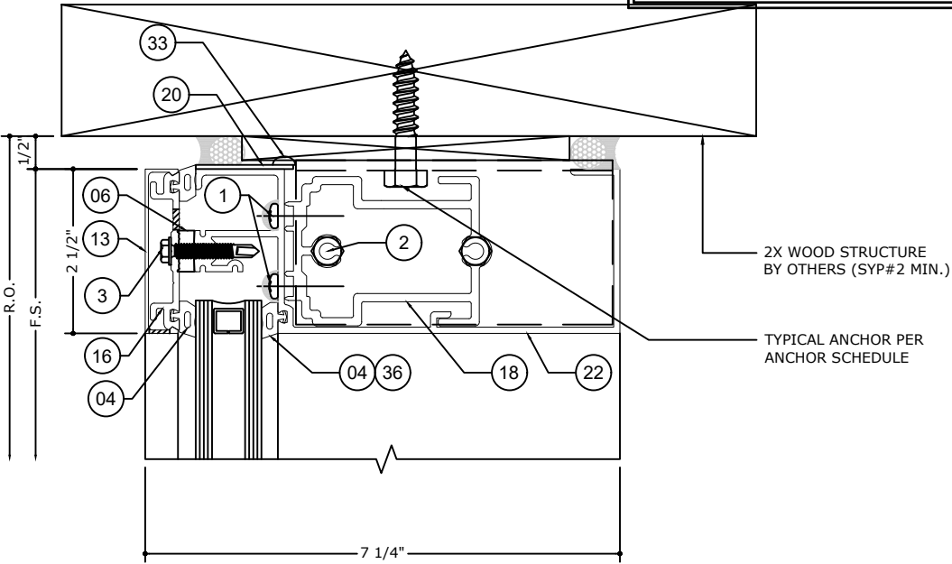
1.1 HEAD DETAIL SCALE: 6" = 1'-0"
