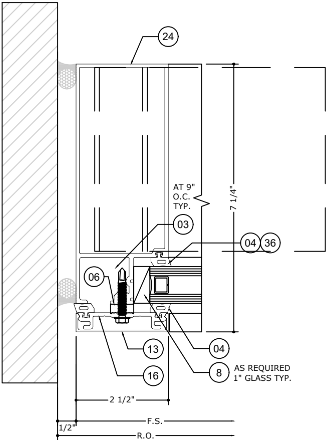
4 JAMB DETAIL SCALE: 6" = 1'-0"
