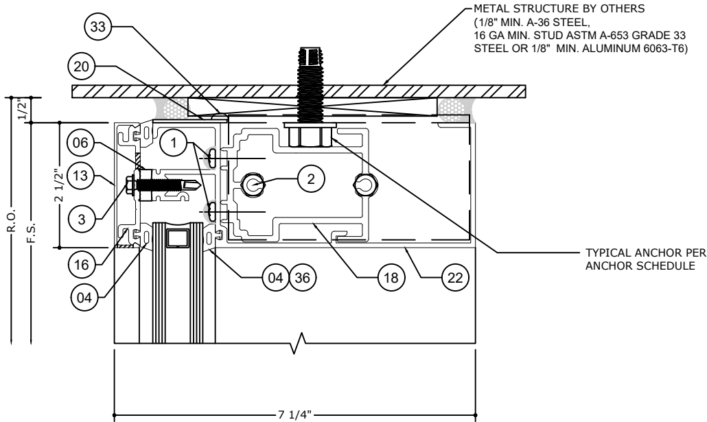
1.2 HEAD DETAIL SCALE: 6" = 1'-0"
