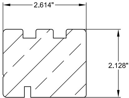
1 FRAME HEAD/JAMB F41-0006_1 WOOD
