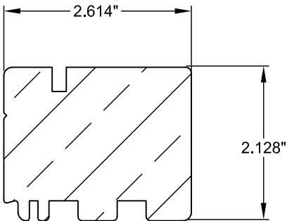
2 FRAME BOTTOM F41-0019 WOOD
