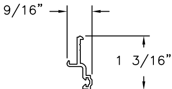
DOOR STOP S46534 ALUMINUM 6063-T6 .070" THICK
