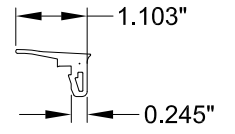
38 E33-1001 SASH GASKET EPDM 70 DUR.
