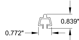
44 E33-0009 SLIDE RAIL ALUMINUM 6060-T66
