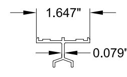
43 E33-0007 GUIDE RAIL ALUMINUM 6060-T66
