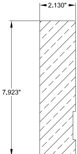
2 F33-0002 FRAME FIXED JAMB WOOD G.50
