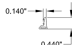
42 E33-1005 SASH GASKET EPDM 70 DUR.
