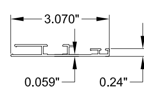
35 E51-0002 SIDE CLAD 110 ALUMINUM 6060-T66
