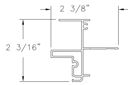
FIN FRAME JAMB CM-18510 ALUMINUM 6063-T5 .050" THICK
