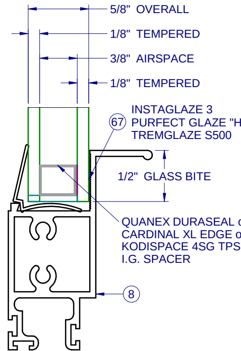
GLASS TYPE B 1:1
