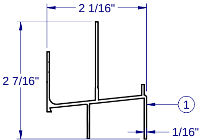
FIN HEAD S-1330
