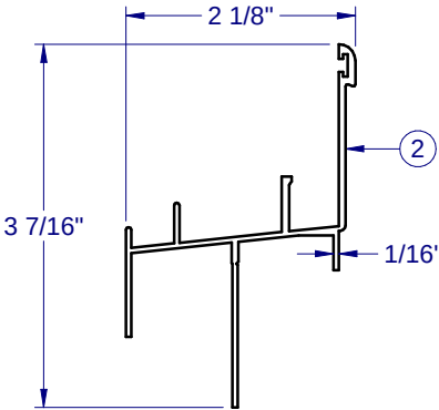
FIN SILL S-1180
