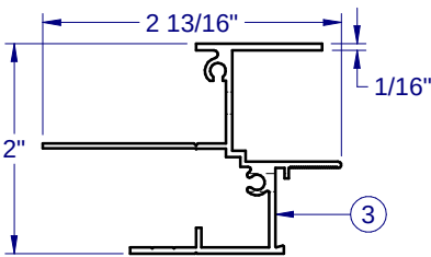
FIN JAMB S-1500
