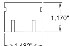
6 DOOR BOTTOM RAIL (PINE SG = 0.42)
