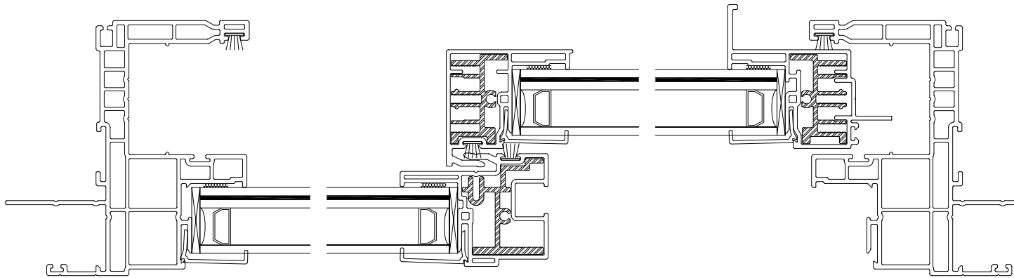
HORIZONTAL CROSS SECTION FIN FRAME
