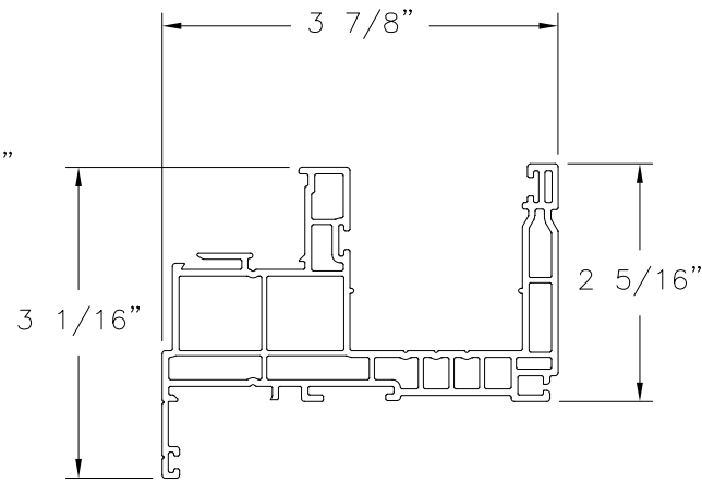
FLANGE FRAME (VM-2363) PVC
