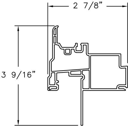
MAIN FRAME (V3823) FIN INSTALLATION RIGID PVC
