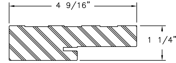
JAMB COMPOSITE
