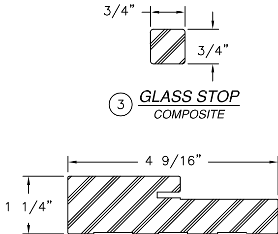
1 JAMB COMPOSITE
