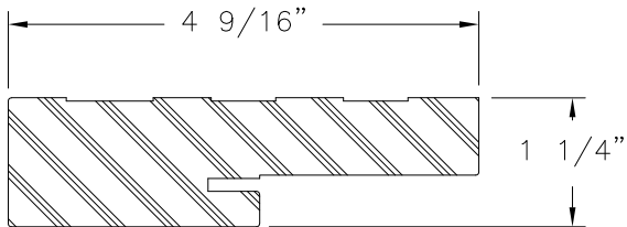
2 JAMB COMPOSITE
