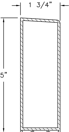
HINGE STILE ALUMINUM 6063-T5 (MS500)
