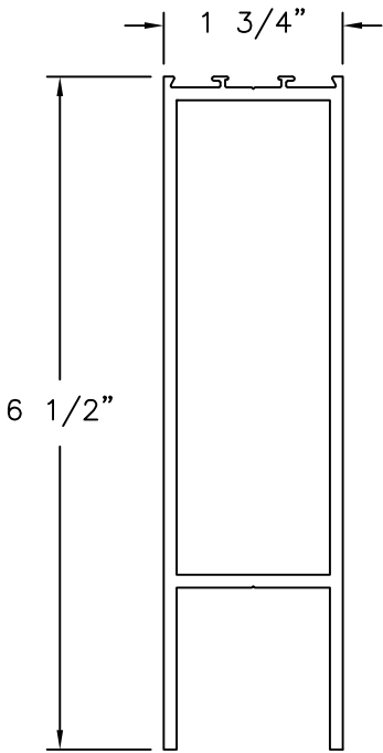
BOTTOM RAIL ALUMINUM 6063-T5 (WS100)
