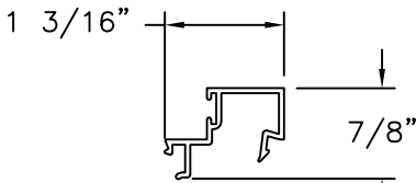
DOOR GLAZING STOP ALUMINUM 6063-T5 (DS040)
