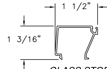
GLASS STOP ALUMINUM 6063-T5 (IM-453)
