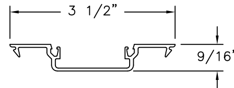
INT. VERT. FILLER ALUMINUM 6063-T5 (IS200)
