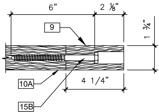
5 6 SECTION SCALE: 1/4" = 1"
