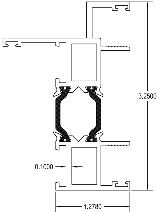
2 P.O. MASTER FRAME - 3 1/4" SCALE 1:1
