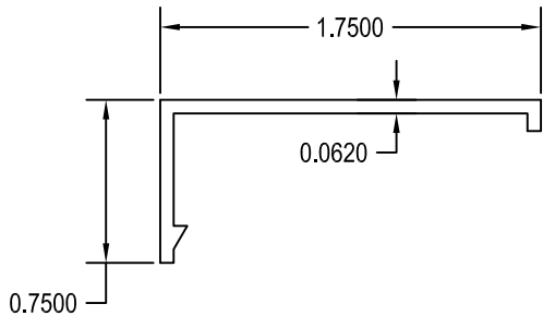
3 #30 TRIM SCALE 1:1
