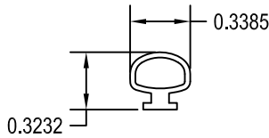
14 FRAME / VENT GASKET SCALE 1:1
