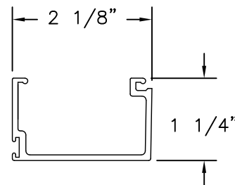
61 DOOR STOP EXTRUDED ALUMINUM 6063-T5 .085" THICK
