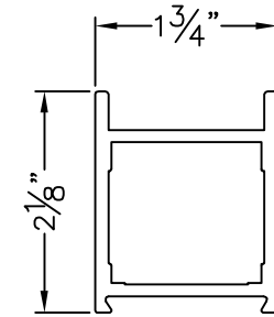
ITEM 6 - E1375 TOP RAIL ~ NARROW STILE
