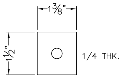
ITEM 16 DOOR ROD WASHER
