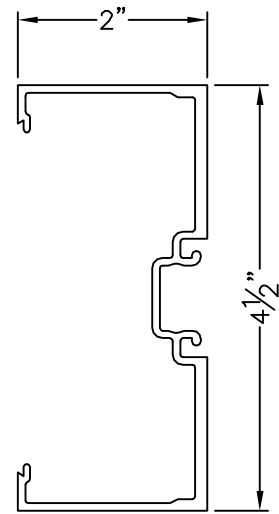
ITEM 1B - E14144 OPEN BACK DOOR JAMB
