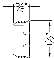
ITEM 14 - E0998 DOOR LUGS
