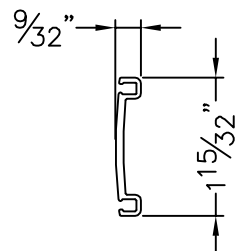
ITEM 10 - E1152 ASTRAGAL
