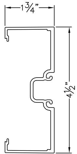
ITEM 1A - E4544 OPEN BACK DOOR JAMB
