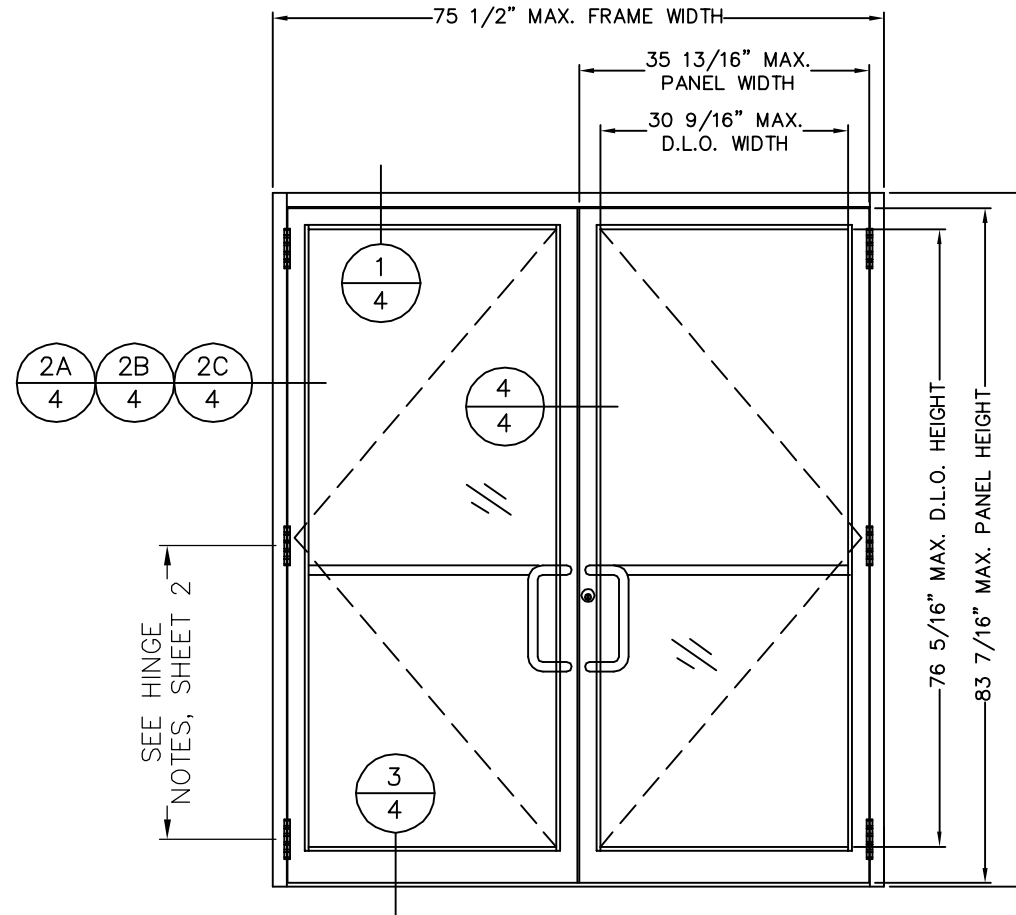
ELEVATION A
