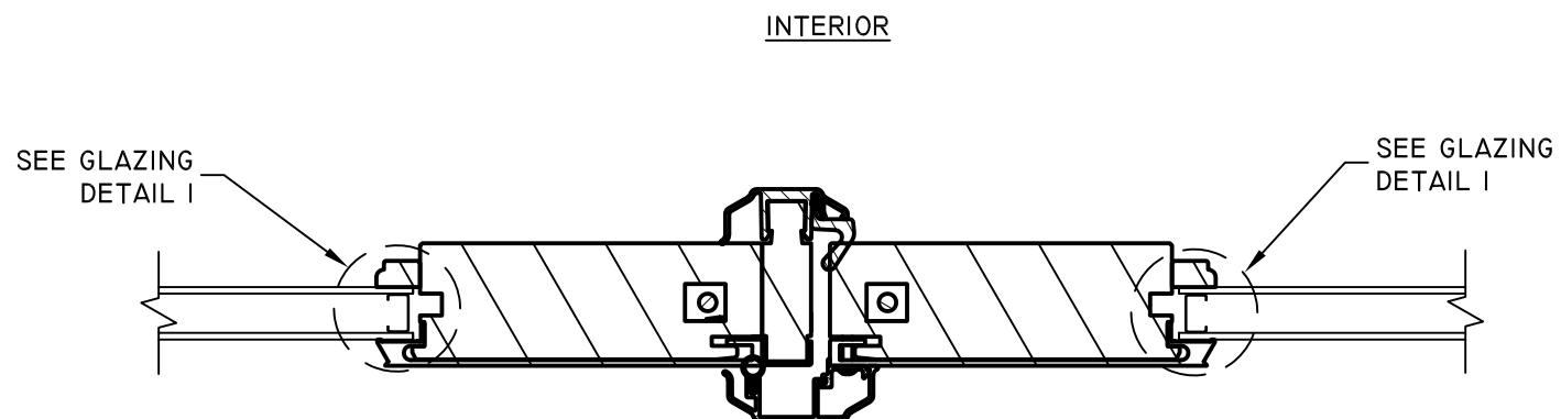
C 4 HORIZONTAL SECTION JAMB
