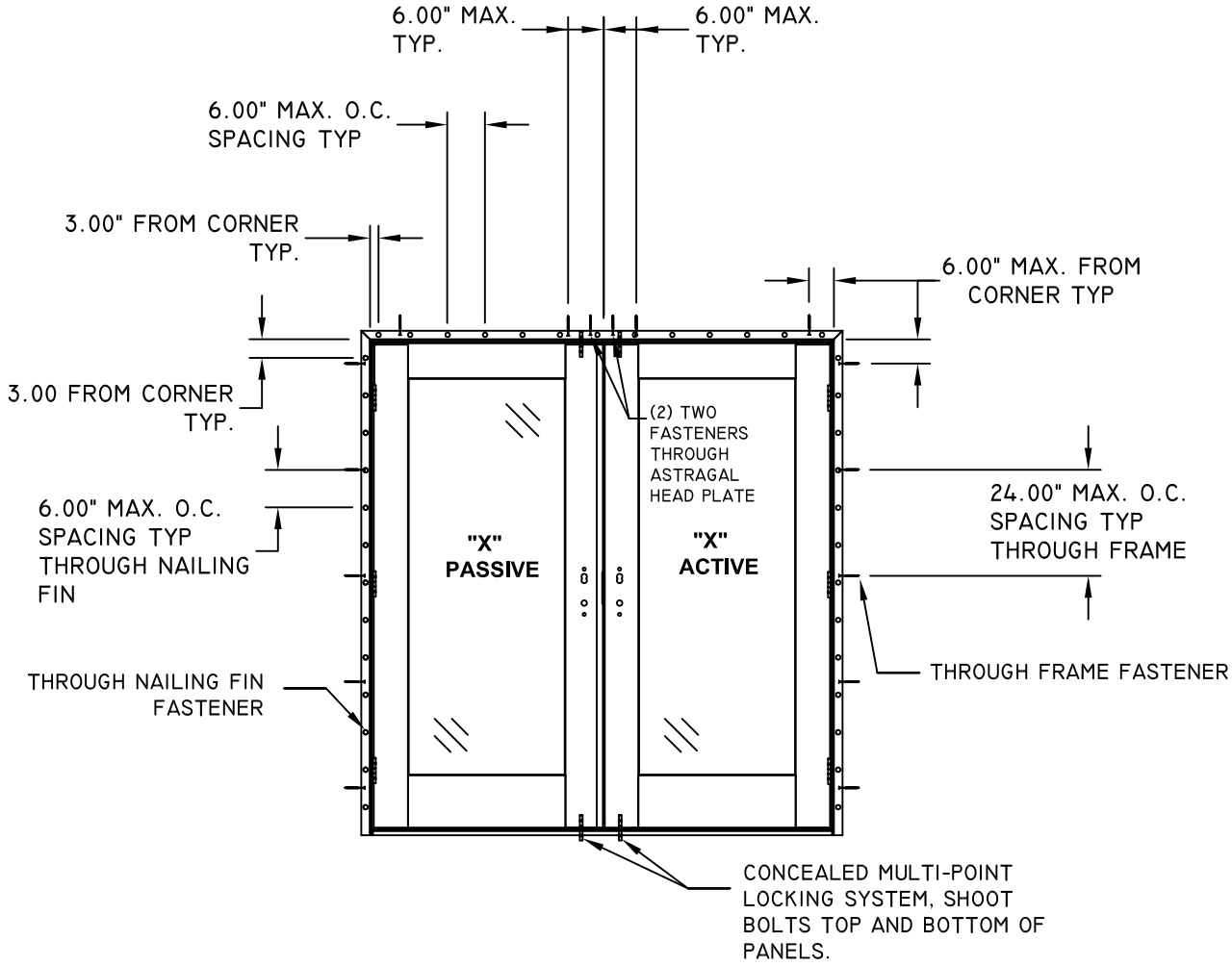
ANCHOR LAYOUT FIN
