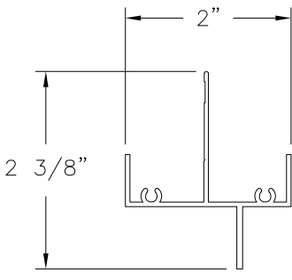
MAIN FRAME FIN INSTALLATION ALUMINUM 6063-T5 (CM-18522)
