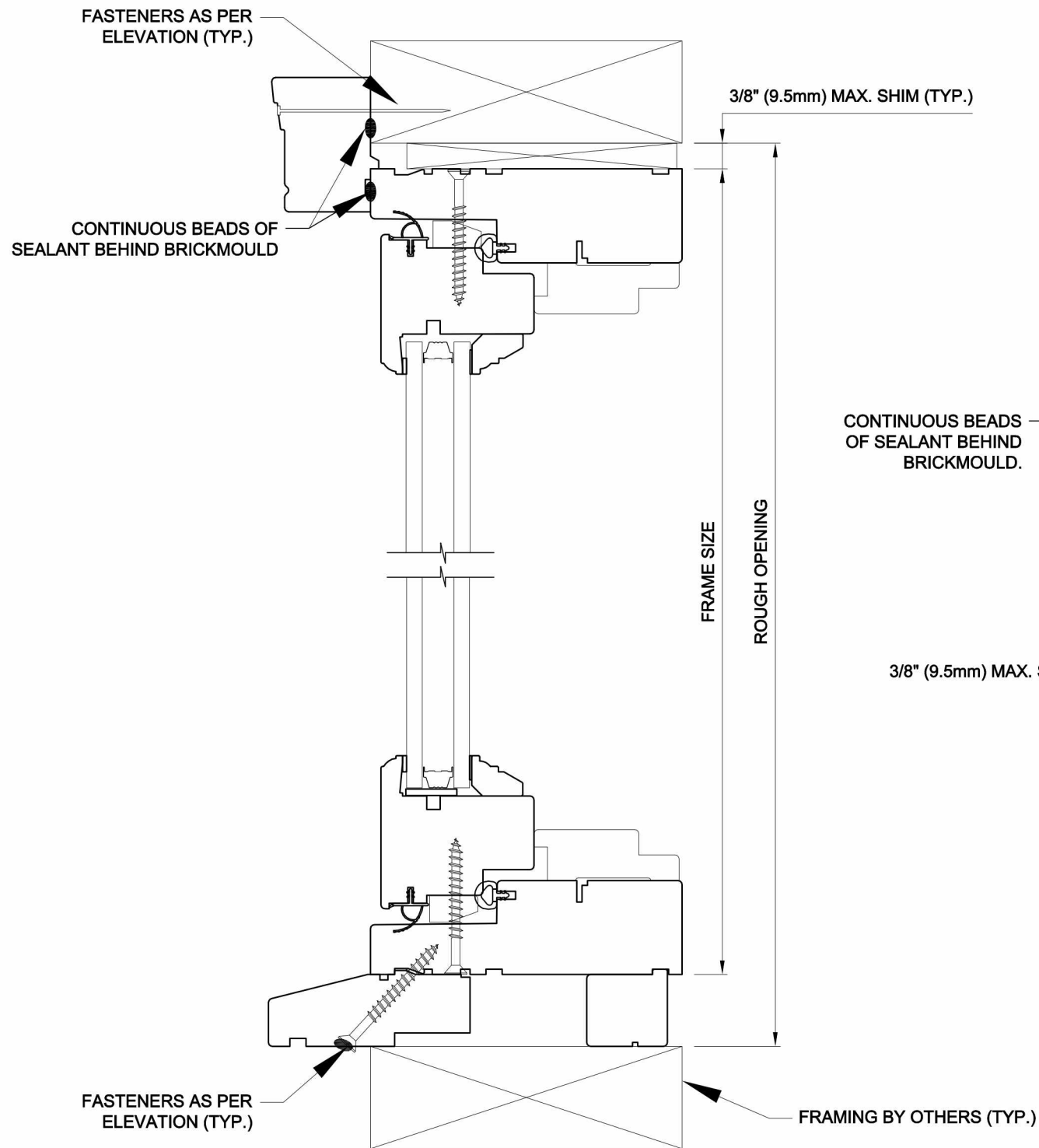
A2 SECTION 1 SCALE: 1:1
