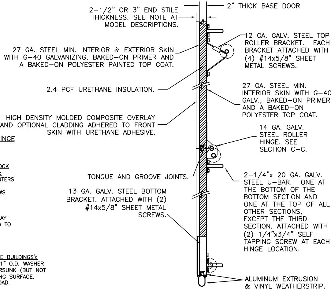
SECTION A-A
