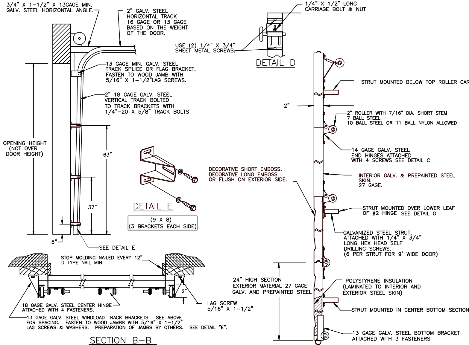
SECTION A-A
