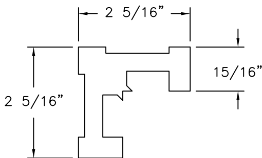
GUSSET ALUMINUM 6063-T6
