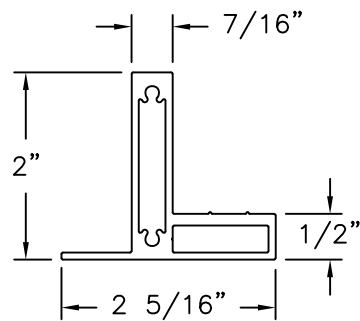
HEAD, SILL & JAMB ALUMINUM 6063-T5 (TAP-950)
