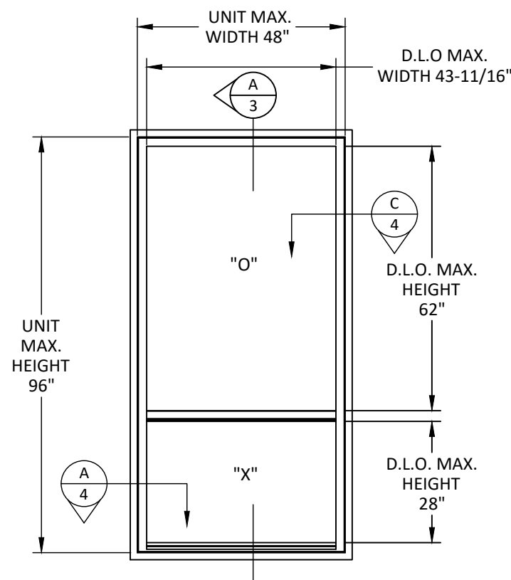
ELEVATION ORIEL
