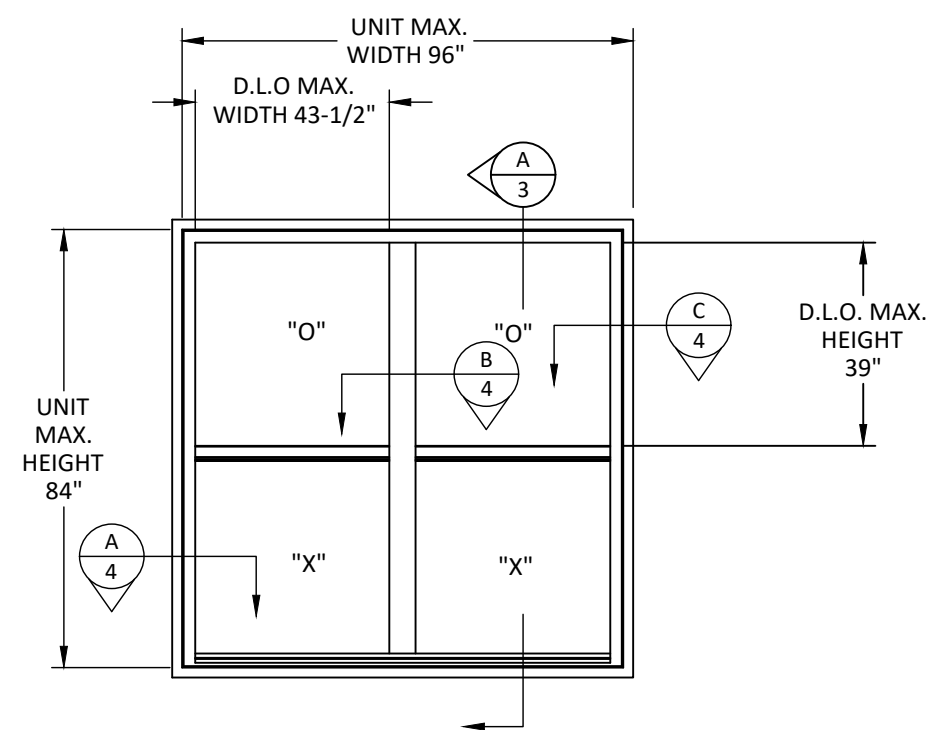
ELEVATION
