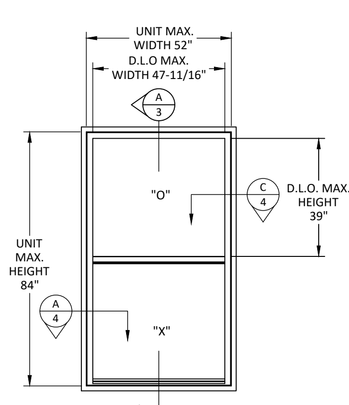
ELEVATION
