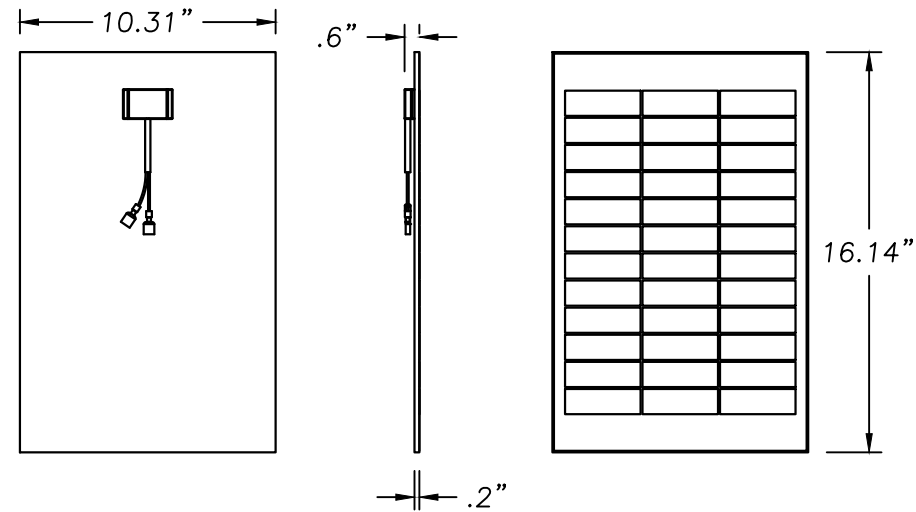
4 RM-1500 SOLAR PANEL
