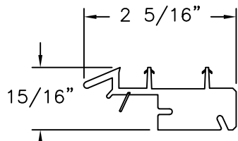
DOOR BOTTOM FOAM & RIGID PVC
