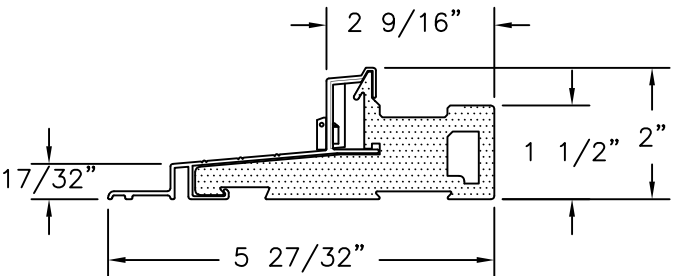
DOOR SILL
