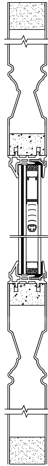
W/MINI-BLIND
