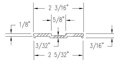
CAP EXTRUSION (H-RC)
