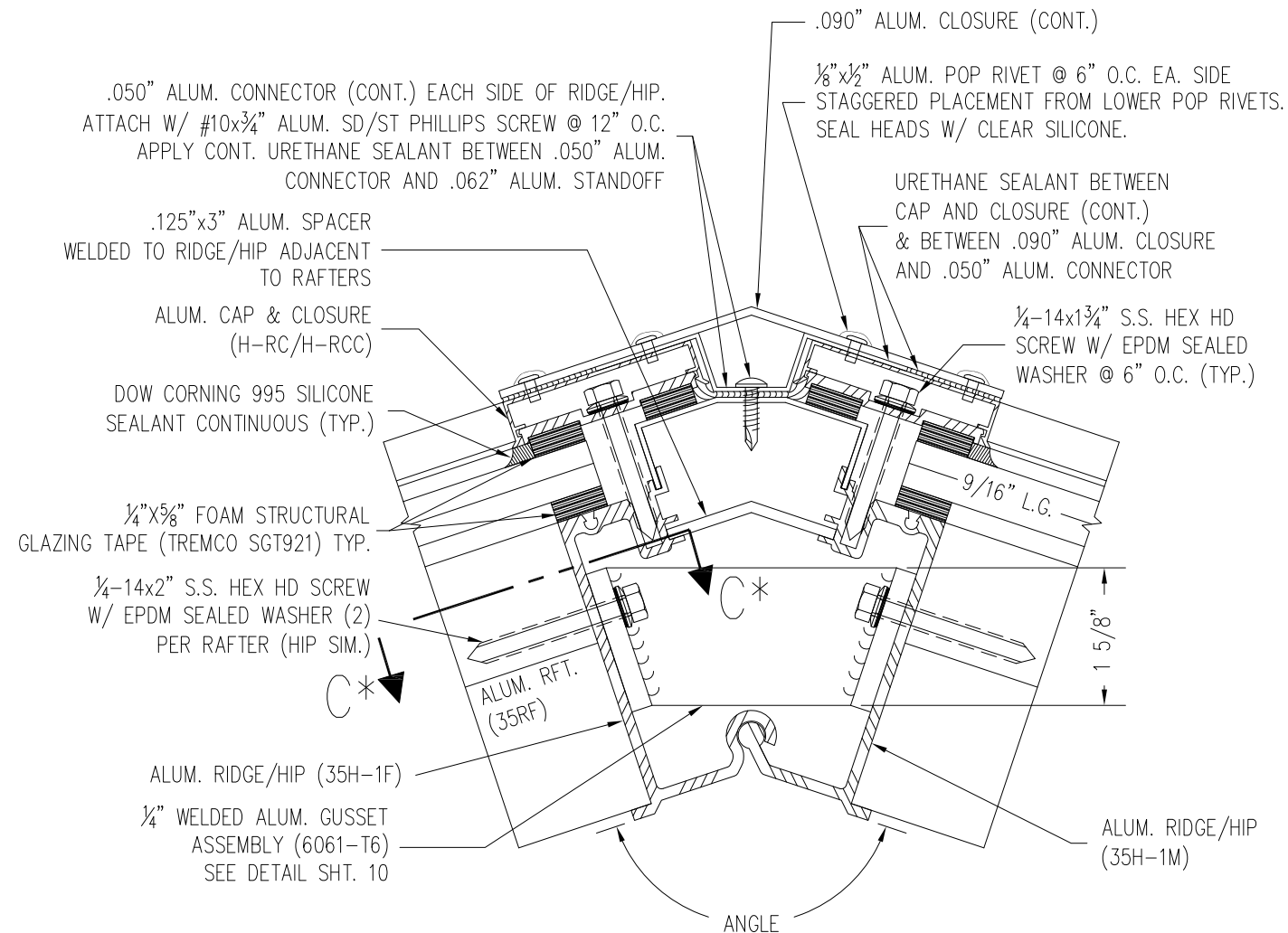
3C RIDGE SECTION - (ANGLE - 143°7'45") SCALE: 6"=1'-0"
