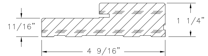
FRAME WOOD G.46 MIN.
