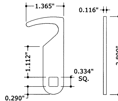
24 LOCKING ARM N.T.S. 410 STAINLESS STEEL
