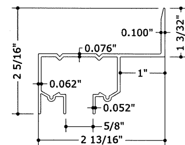
38 ALT. WALL HEADER N.T.S. 6063-T6
