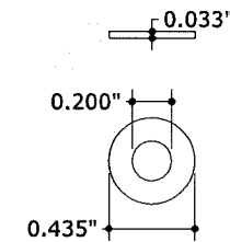
21 WASHER N.T.S. STAINLESS STEEL
