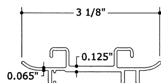
30 HIGH IMPACT CENTERMATE INSERT N.T.S. 6063-T6
