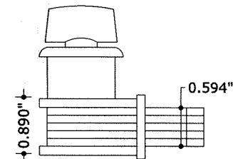
34 HOOK BOLT DEAD LOCK N.T.S. ALUMINUM
