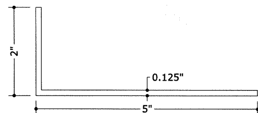
27 2"x5"x0.125" ANGLE N.T.S. 6063-T6
