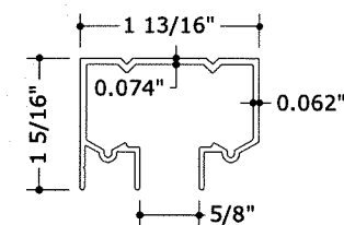
37 ALT. CEILING HEADER N.T.S. 6063-T6
