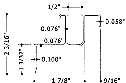
15 WALL SILL TRACK N.T.S. 6063-T6
