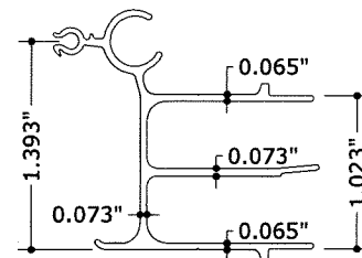
4 MALE CENTERMATE N.T.S. 6063-T6
