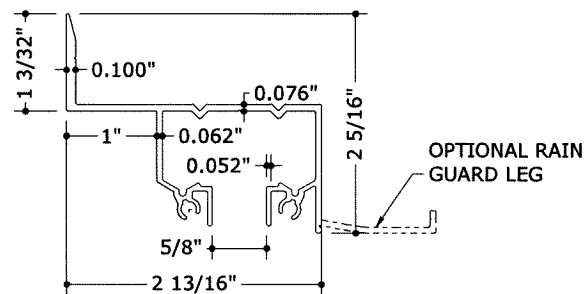
10 WALL HEADER N.T.S. 6063-T6
