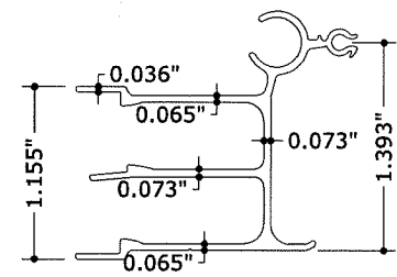
5 FEMALE CENTERMATE N.T.S. 6063-T6
