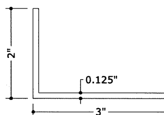
36 2"x3"x0.125" ANGLE N.T.S. 6063-T6
