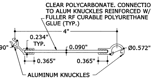
2 WINDOW BLADE N.T.S. 6063-T6/POLYCARBONATE
