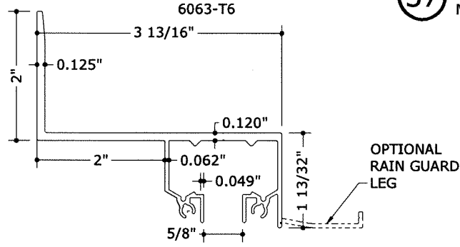
13 BUILD-OUT WALL HEADER N.T.S. 6063-T6
