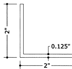
35 2"x2"x0.125" ANGLE N.T.S. 6063-T6
