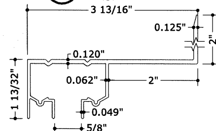
39 ALT. BUILD-OUT WALL HEADER N.T.S. 6063-T6
