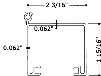
29 HIGH IMPACT CENTERMATE N.T.S. 6063-T6
