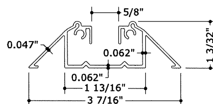
16 WALKOVER TRACK N.T.S. 6063-T6
