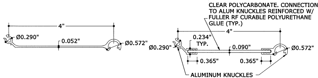
1 STANDARD BLADE N.T.S. 6063-T6
