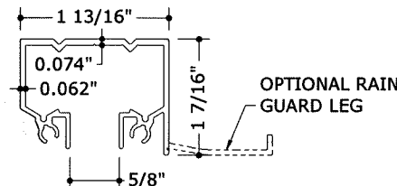
9 CEILING HEADER N.T.S. 6063-T6
