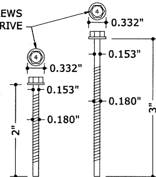
20 KNUCKLE SCREWS N.T.S. STAINLESS STEEL
