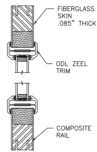
OPTION 41 ODL ZEEL TRIM
