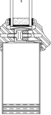
OPTION 8 PLUGLESS TRIM W/TAPE
