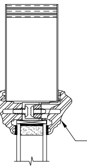
PLUGLESS TRIM
