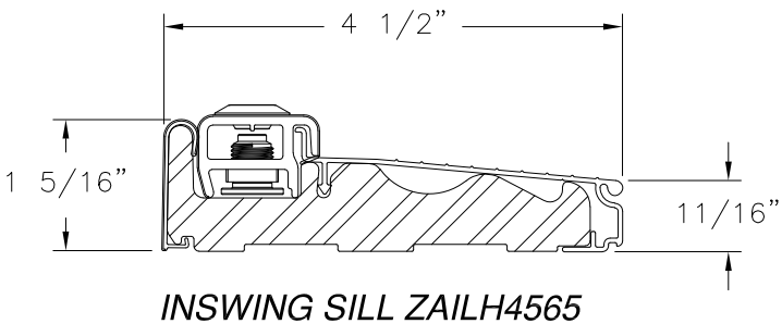
INSWING SILL ZAI4565F
