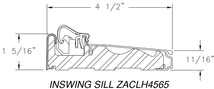
INSWING SILL ZAC4565F
