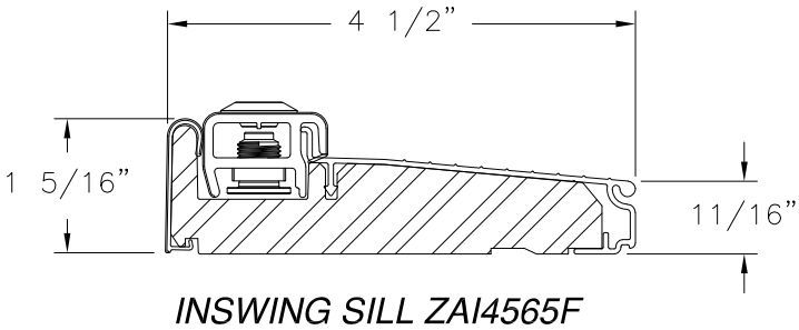
INSWING SILL ZAIL4565
