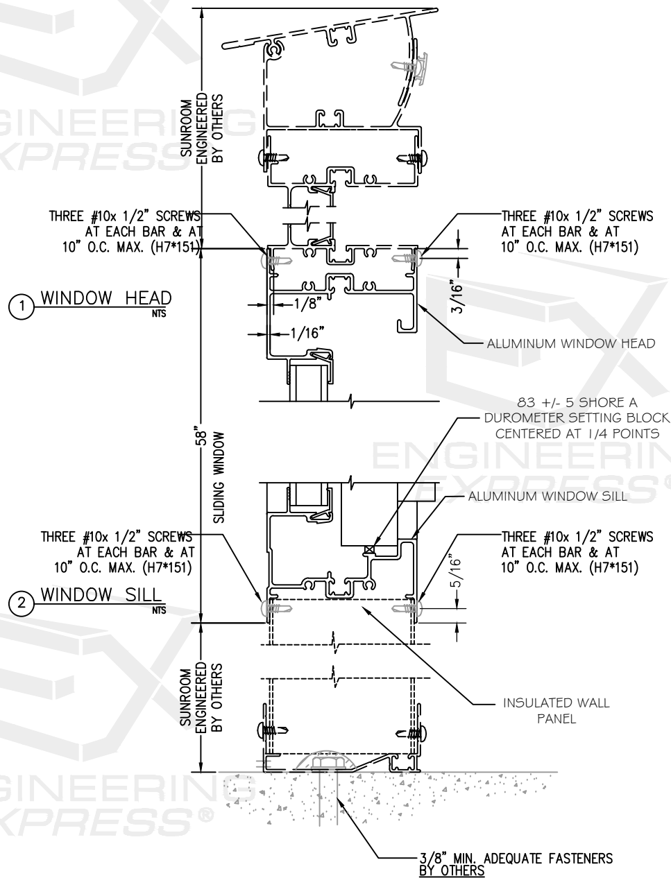
SECTION B-B SCALE: NTS
