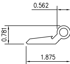
14 5 1/4" HINGE
