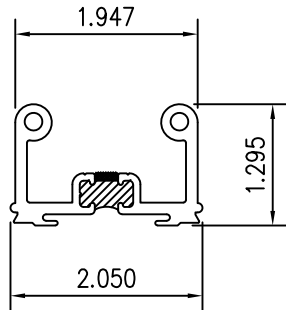
4 FRAME LUG
