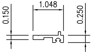
3 FRAME CAP
