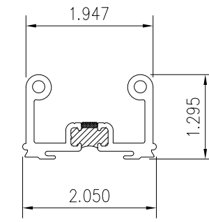
4 FRAME LUG
